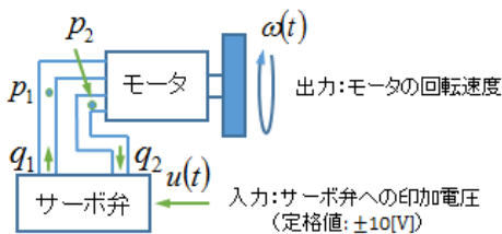
図3 水圧モータシステム
